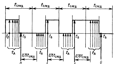
Рис. 2.10. Временные диаграммы сигналов при чтении двухфазного кода
